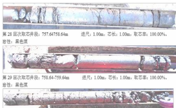
Рис. 3. Образцы керна Fig. 3. Core samples
