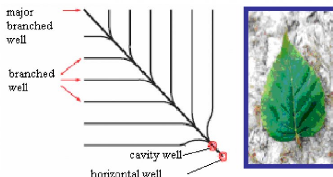
Рис. 4. Многозабойная горизонтальная скважина от CDX Co
