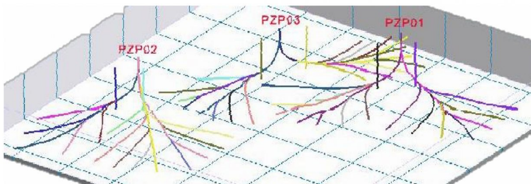
Рис. 5. Группа многозабойных скважин области Паньжунг Fig. 5. A group of multilateral wells area Panjang
