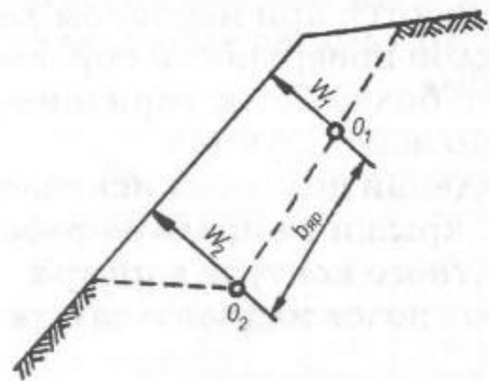
Рис. 4.8. Схема двухъярусного расположения зарядов сброса
