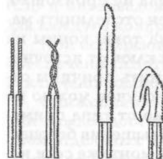
Рис. 2.5. Порядок процесса соединения проводов от двух изделий
