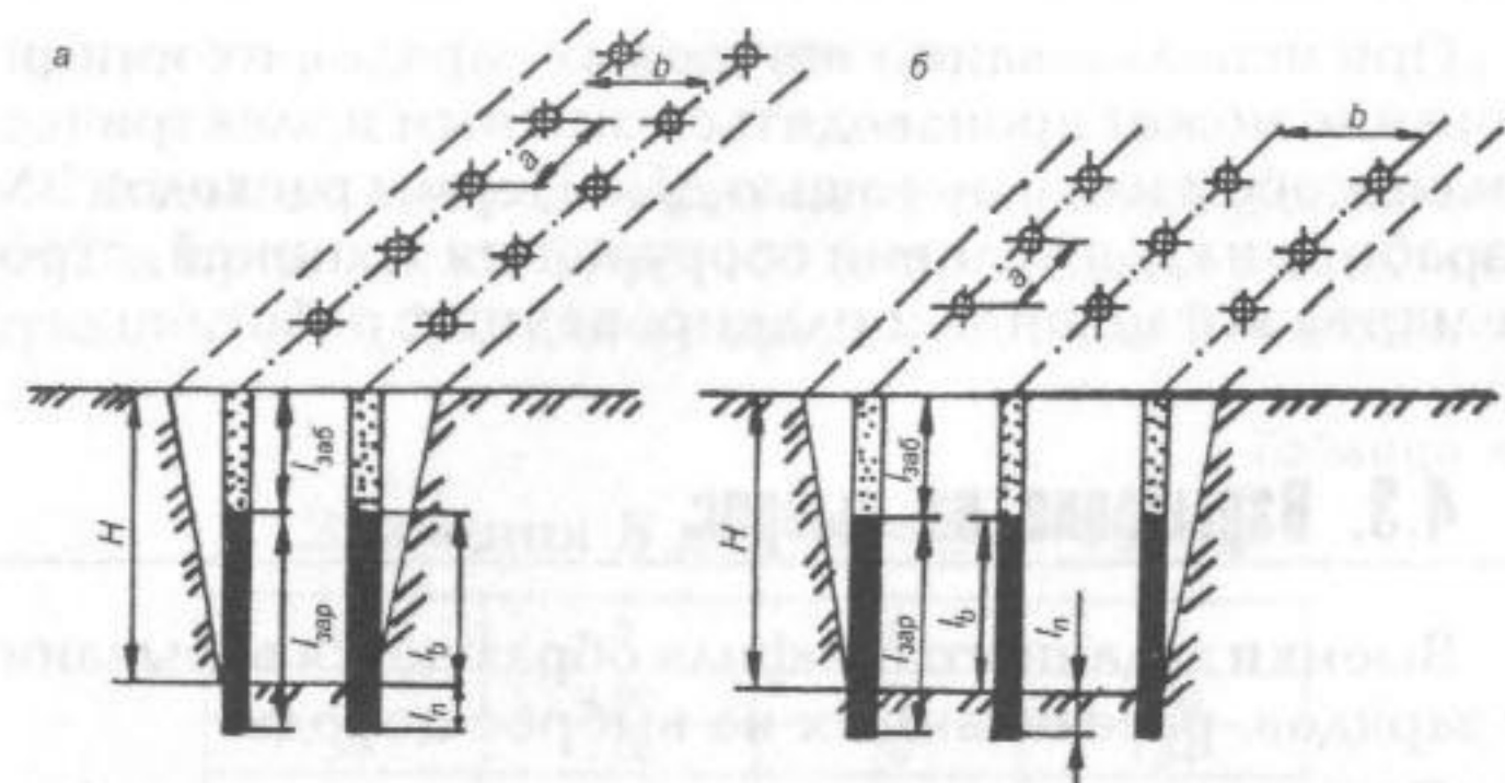
Рис. 4.4. Схема расположения зарядов при сооружении траншей
