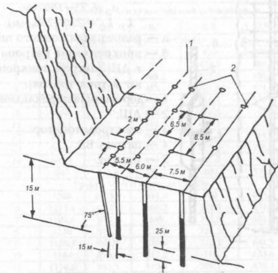
Рис. 4.1. Расположение контурных (1) и отбойных (2) скважин на уступе.
