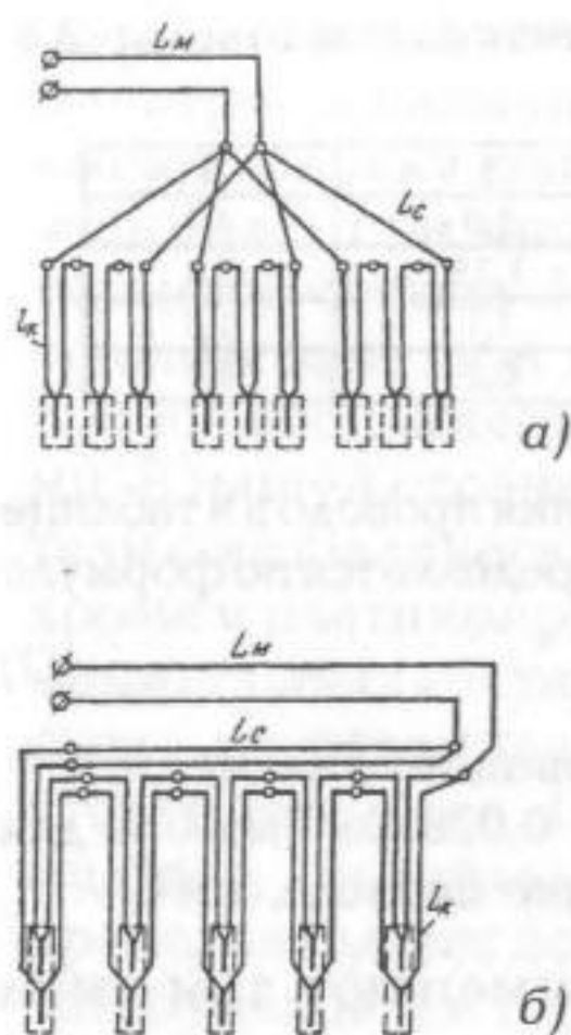
Рис. 2.3. Последовательно-параллельное соединение электродетонаторов: а — в заряд введен один электродетонатор; б — в заряд введены два электродетонатора.
