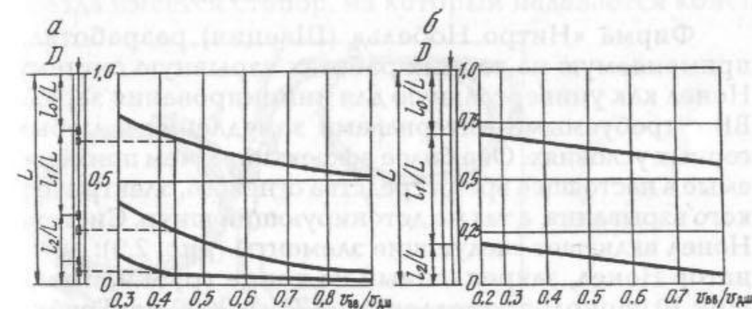
Рис. 2.8. Номограмма для определения местоположения промежуточных детонаторов в заряде, сформированном из однотипных ВВ:
