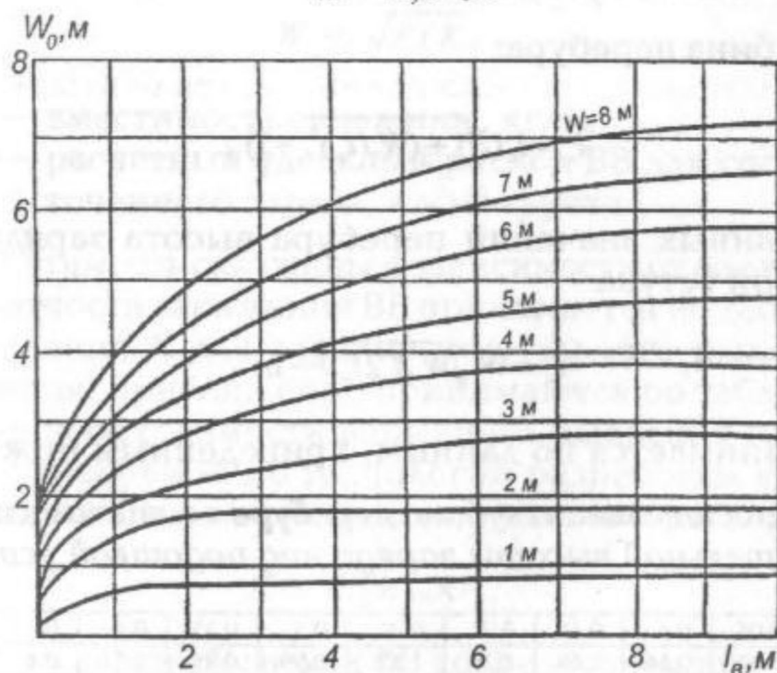
Рис. 2.4. Зависимость величины преодолеваемого сопротивления по подошве уступа W_0 от длины заряда над подошвой уступа l_0 при взрывании скважинных зарядов без перебура
