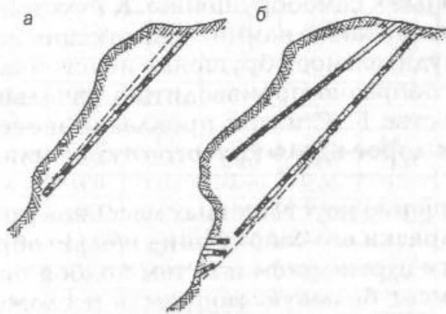
Рис. 4.9. Расположение скважин для обрушения неустойчивых массивов малой (а) и большой (б) мощности.
