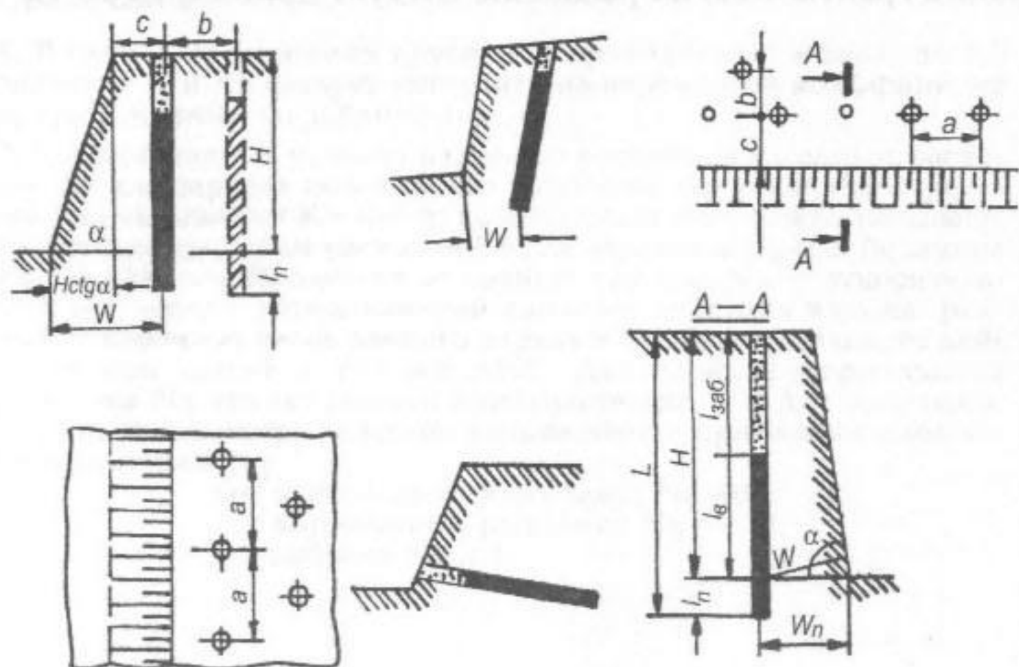
Рис. 2.1. Схемы расположения шпуровых зарядов
