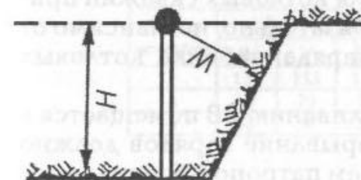
Рис. 2.5. Котловой заряд
