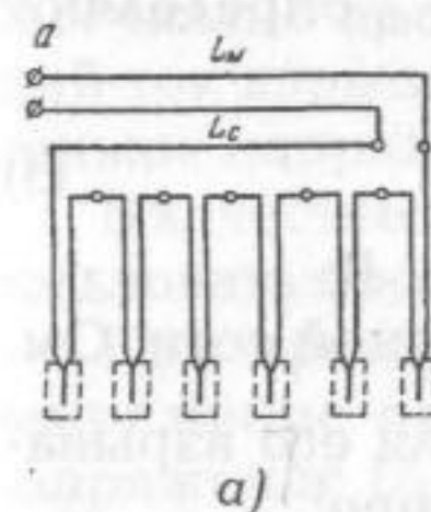
Рис. 2.2. Последовательное соединение электродетонаторов: а — в заряд введен один электродетонатор; б — в заряд введены два электродетонатора, четы-концевика выведены из выработки; в — в заряд введены два электродетонатора, на земную поверхность выведены два концевика.
