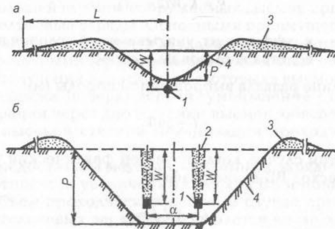
Рис. 4.5. Схема расположения зарядов выброса сосредоточенных (а) и траншейных (б):
