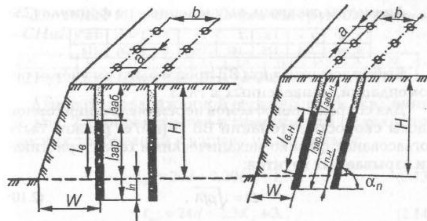
Рис.2.2. Схема расположения вертикальных скважинных зарядов
