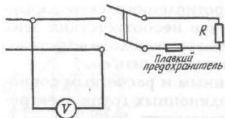
Рис. 2.4. Схема замера падения напряжения в подводящей сети (источнике тока)
