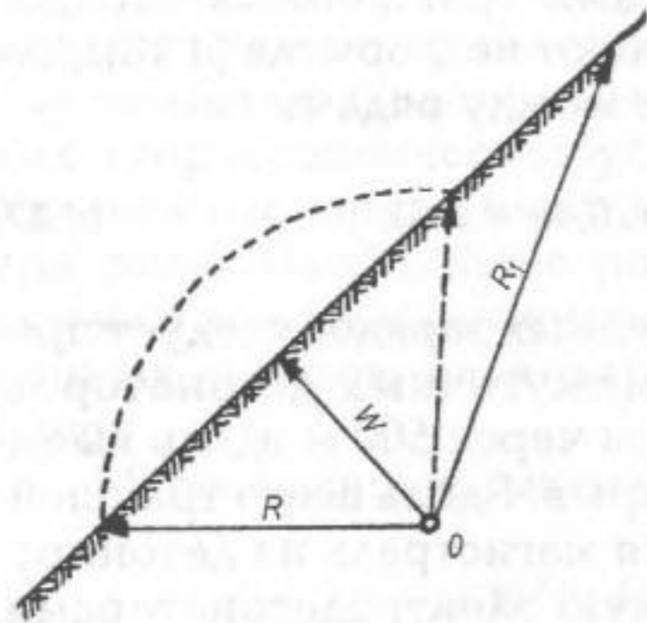
Рис. 4.6. Схема однорядного расположения зарядов сброса
