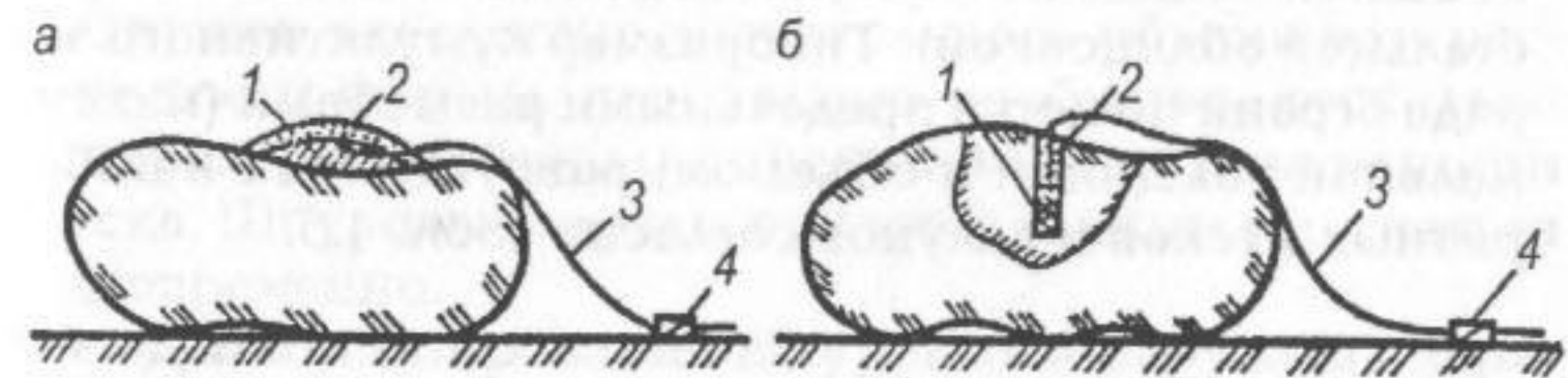
Рис. 4.3. Разрушение негабарита накладными (а) и шпуровыми (б) зарядами:
