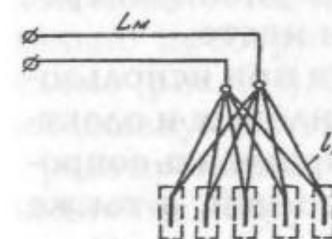
Рис. 2.1. Параллельное соединение электродетонаторов
