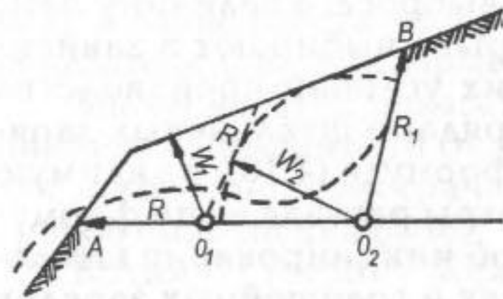
Рис. 4.7. Схема двухрядного расположения зарядов сброса
