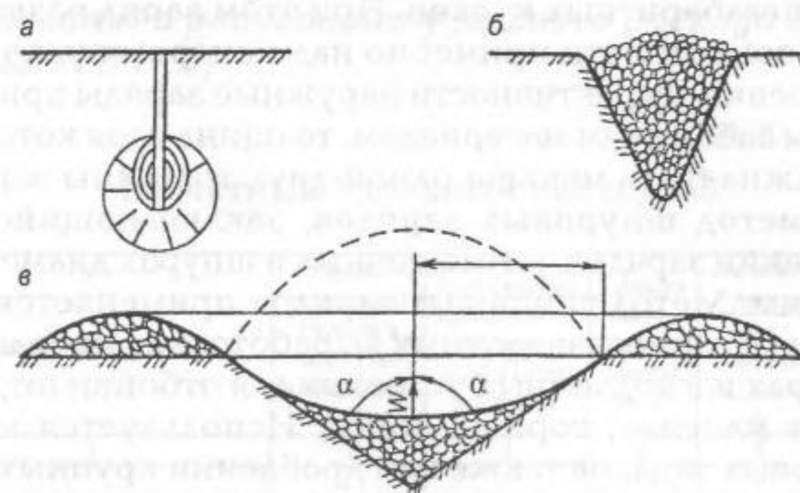
Рис. 1.1. Характер действия взрыва при зарядах камуфлета (а), рыхление (б) и выброса (в)
