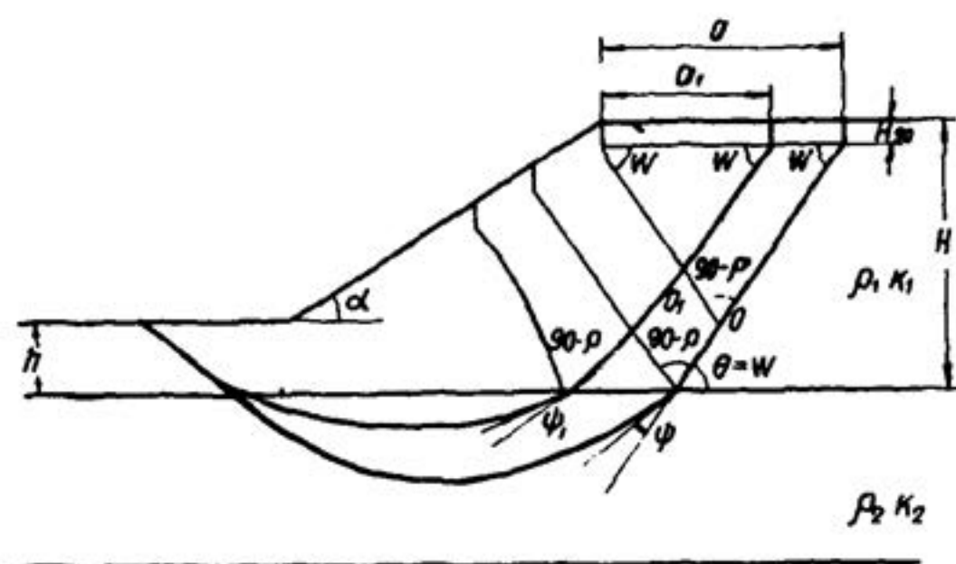
Рис.3. Схема оползня выпирания
