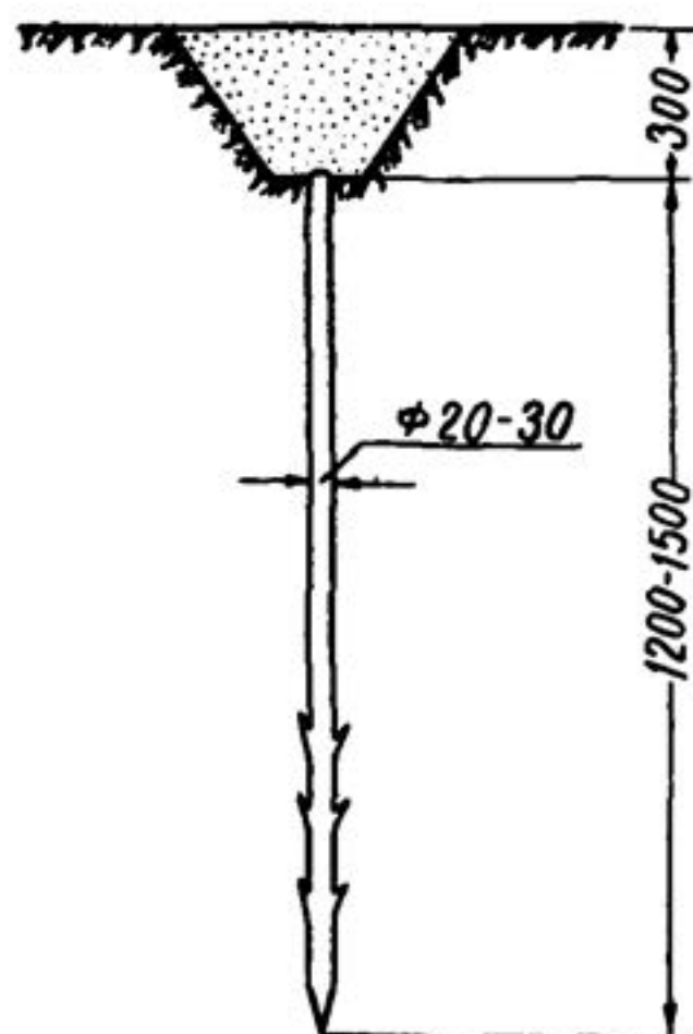
Рис.7. Тип забивного репера
