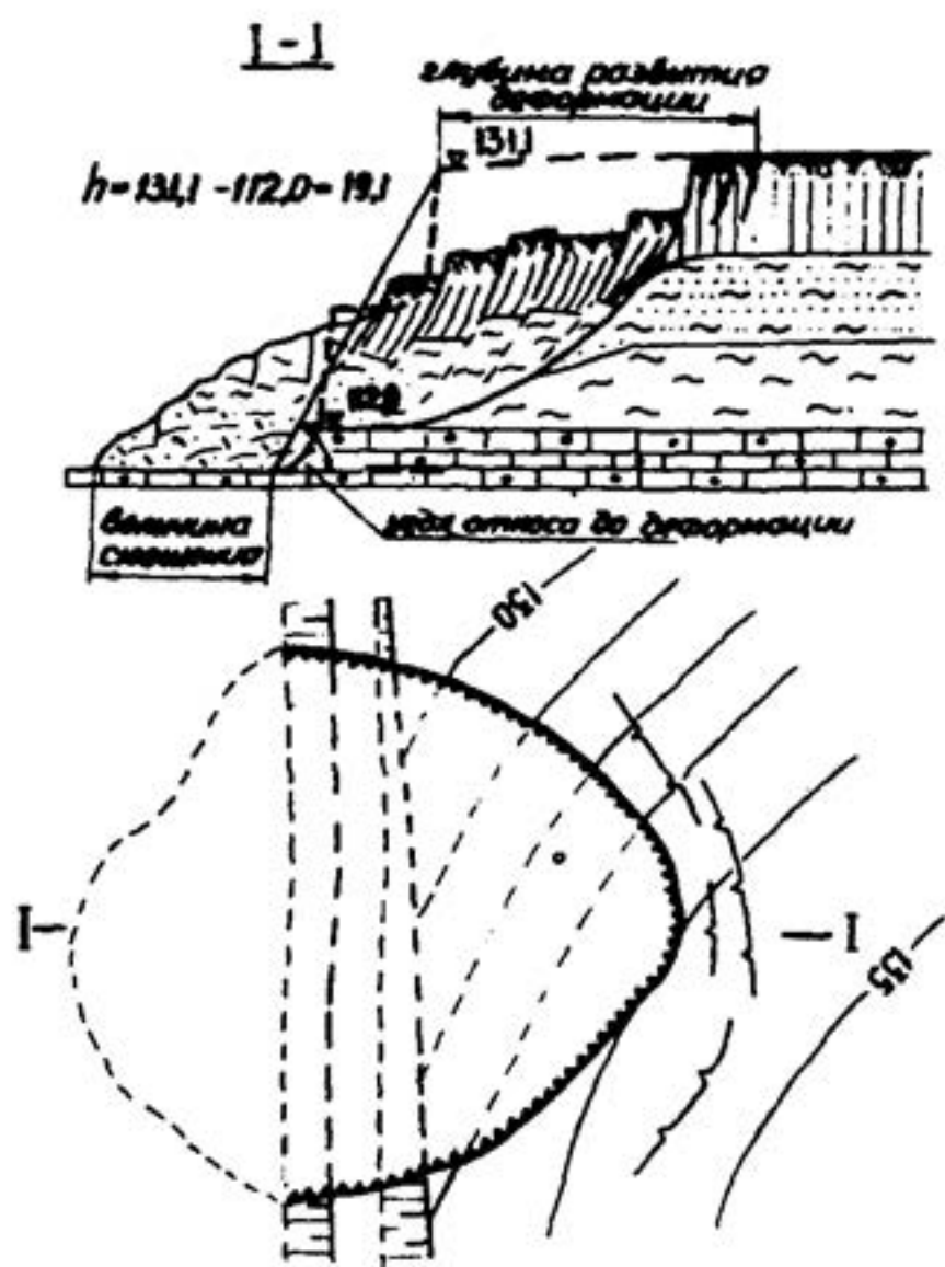
Рис.20. Размеры оползня рабочего борта карьера
