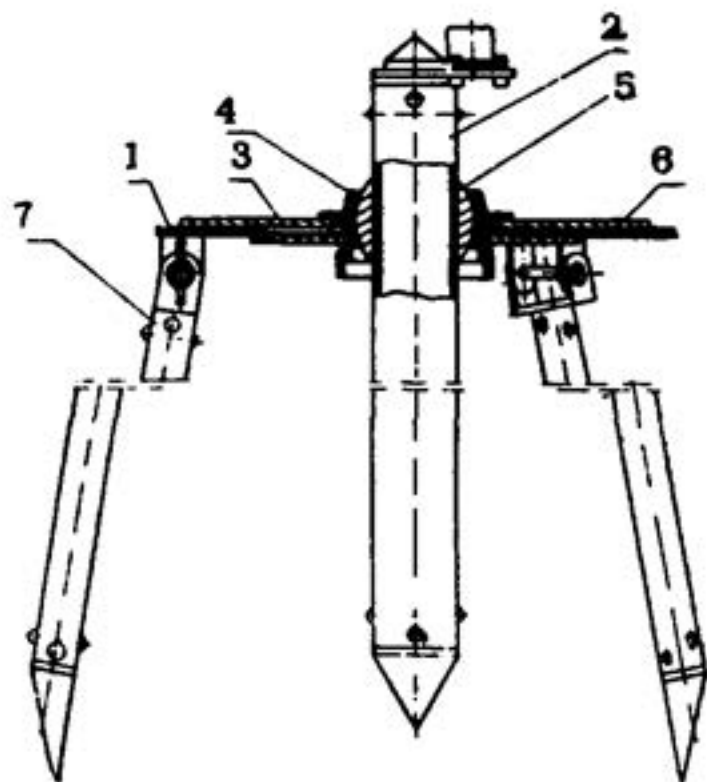
Рис.1. Жесткий отвес ОЖ-3 0.7-0.8 мм.
