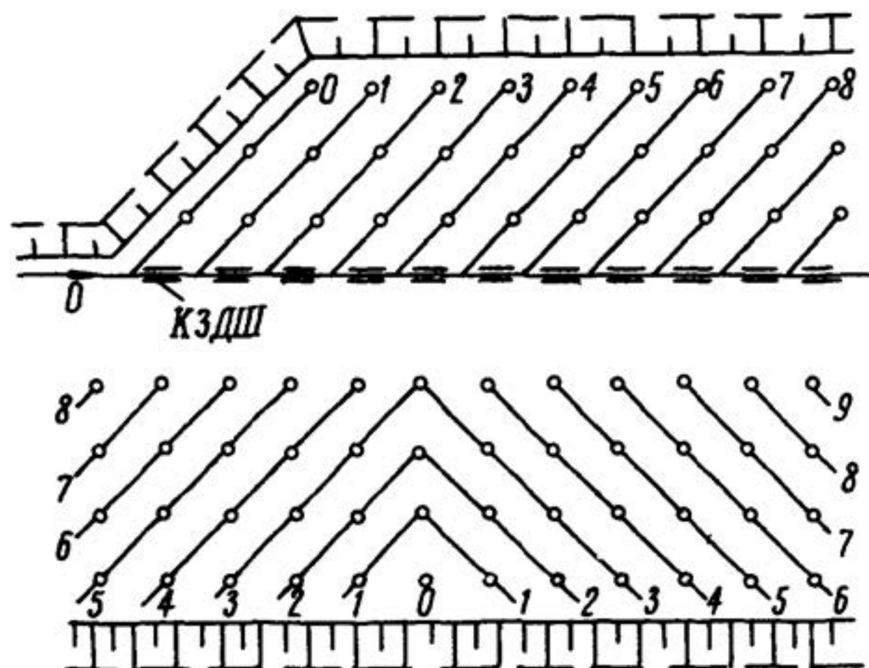
Рис.3. Диагональные схемы короткозамедленного взрывания
