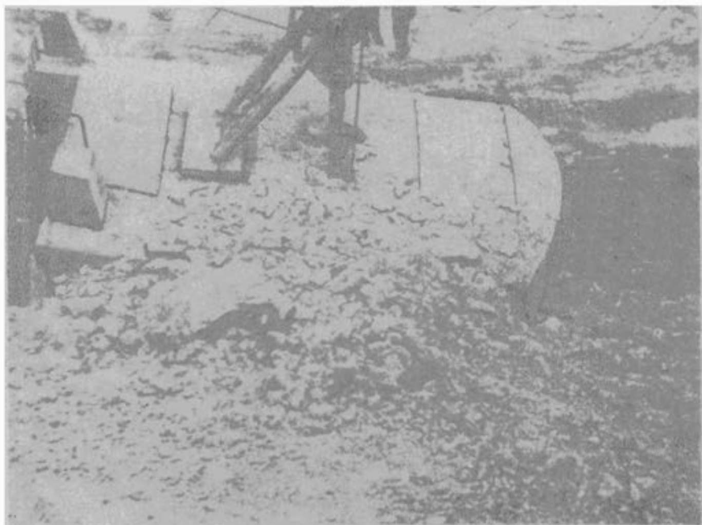
Рис.3. Обрушение уступа 17 августа 1967 года на карьере "Миллионный"
