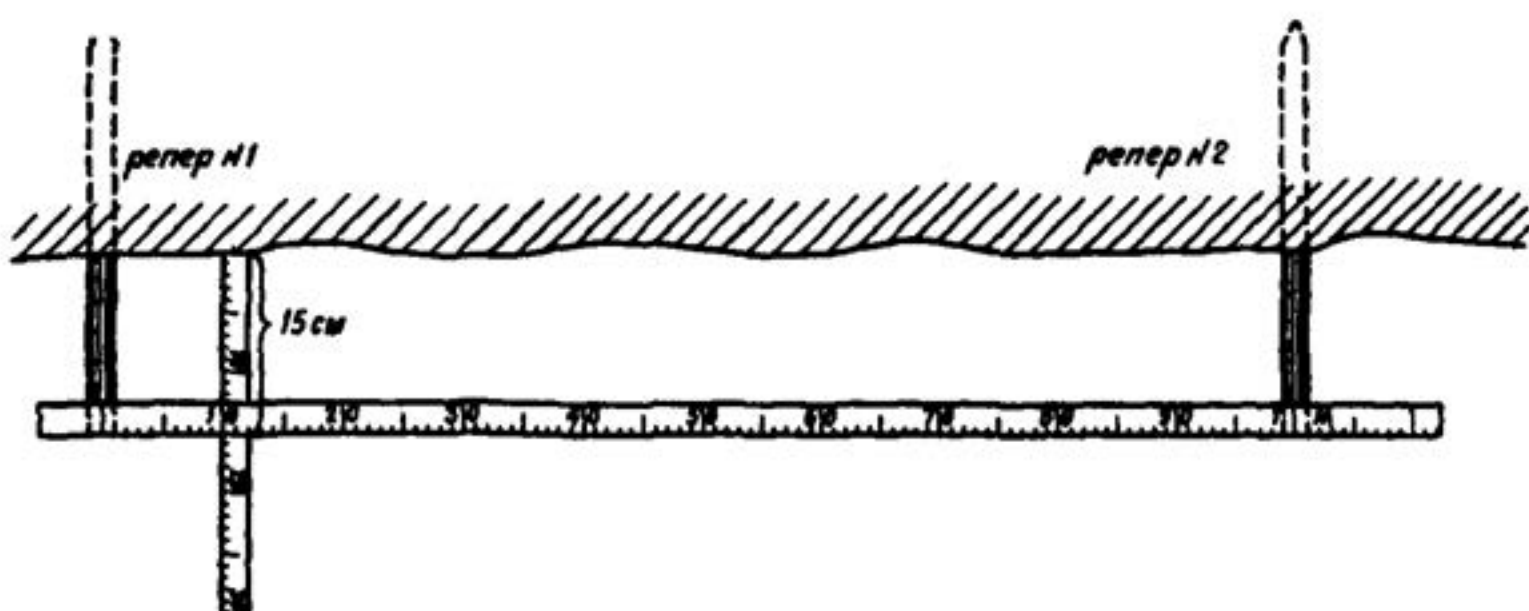
Рис.16. Замер превышений реперов над поверхностью откоса (вид сверху)
