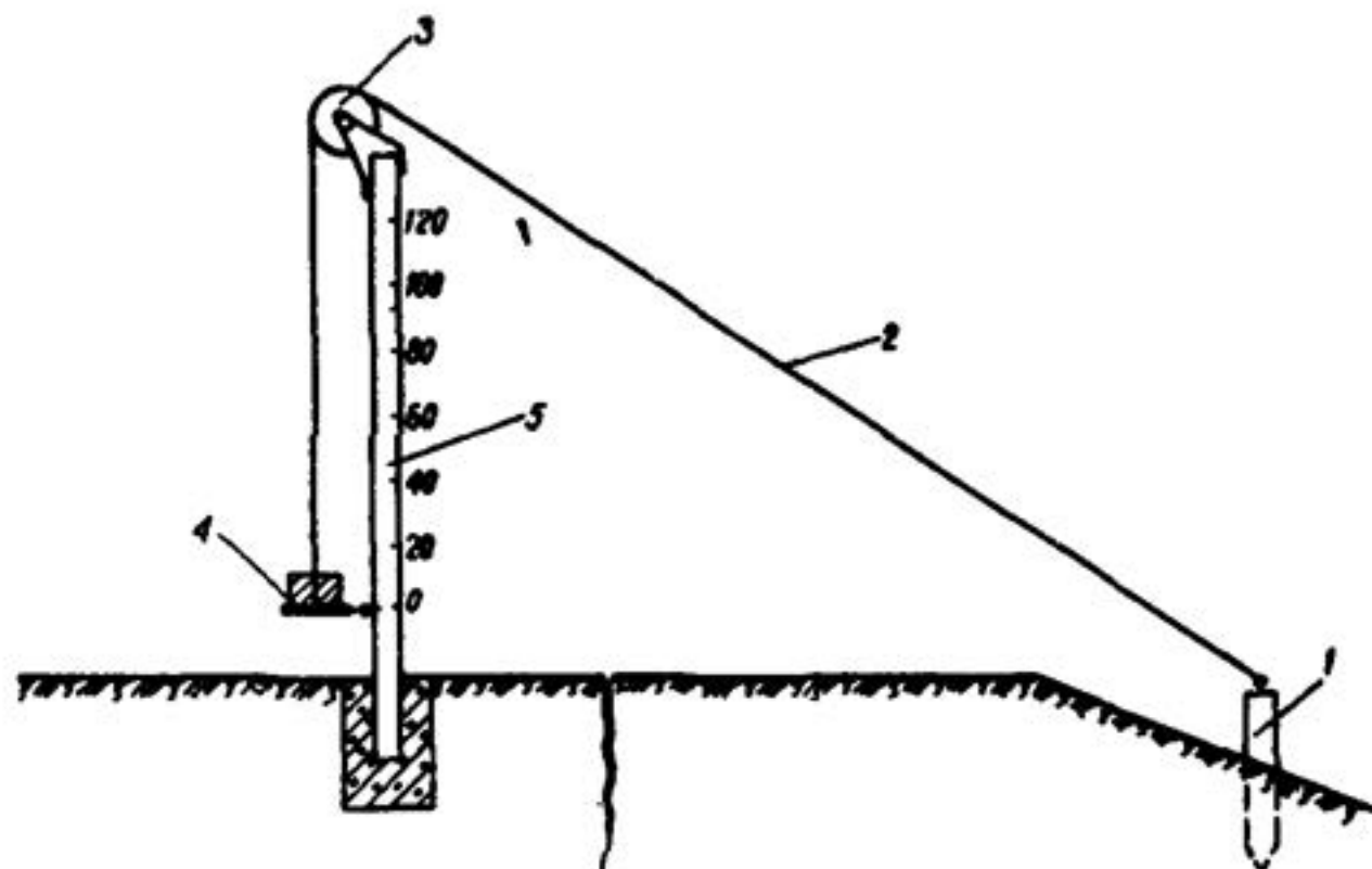
Рис.10. Наблюдения за раскрытием трещины с использованием проволоки и цифрованной рейки
