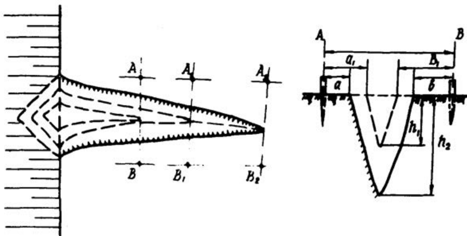
Рис.14. Наблюдения за развитием промоины
