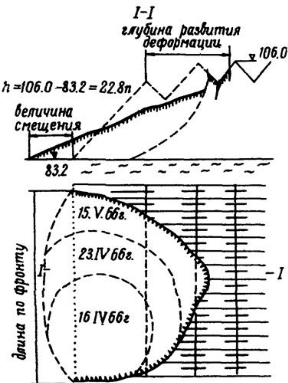
Рис.19. Развитие оползня внутренних отвалов
