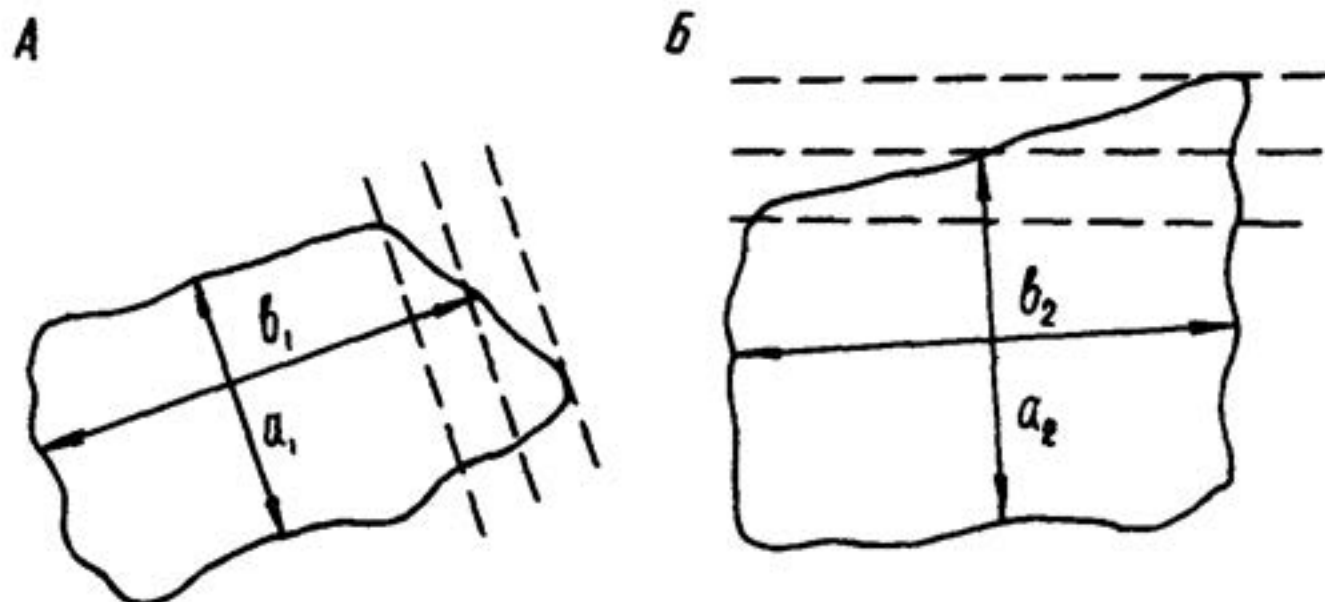
Рис.1. Определение размеров и площади сечения образца (А и Б-верхняя и нижняя грани образца)
