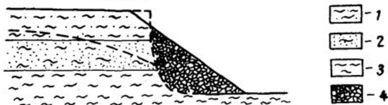
Рис.18. Схема пригрузки фильтрующего песчано-глинистого откоса
