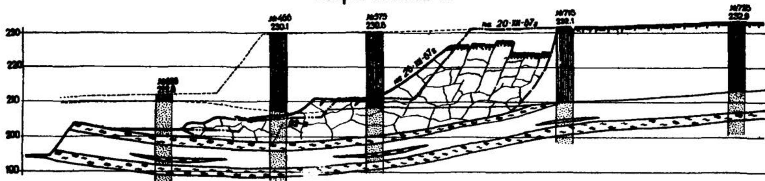
Рис.2. Разрезы плану участка оползня №2 дник "Южный")
