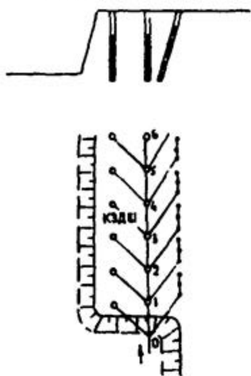
Рис.5. Одновременное взрывание зарядов дробления и отрезной щели
