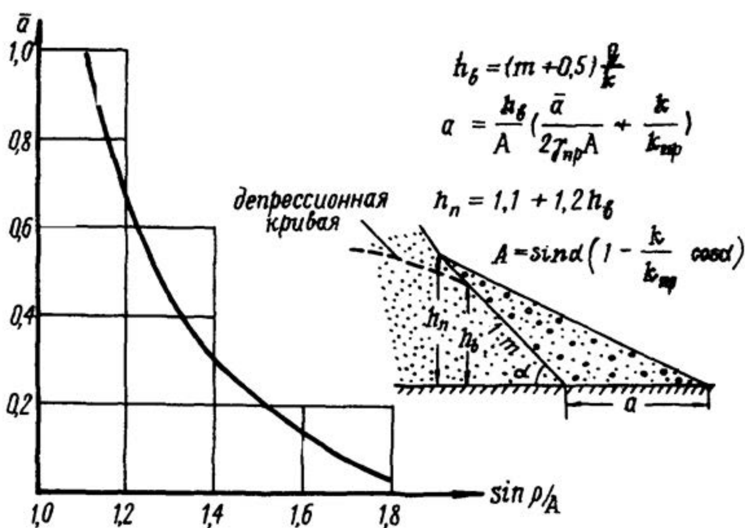
Рис.17. Схема для определения параметров пригрузочной призмы
